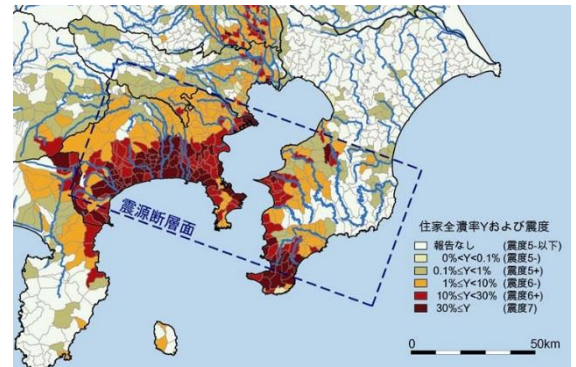
震度分布図
